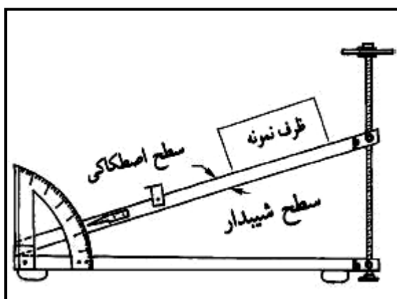
شکل ۲- طرح‌واره وسیله تعیین ضریب اصطکاک استاتیکی
