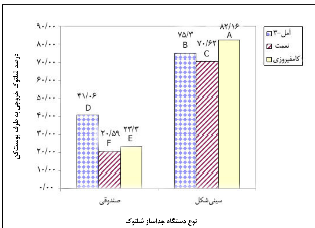
شکل ۳- مقایسه میانگین‌های درصد شلتوک خروجی به طرف پوست‌کن در اثر متقابل نوع دستگاه جدا ساز و رقم شلتوک
