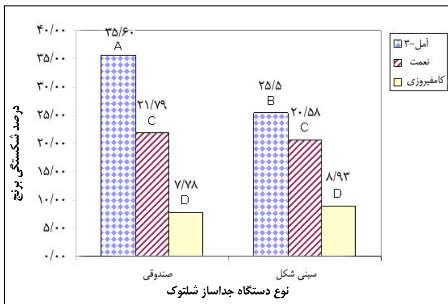
شکل ۵- مقایسه میانگین‌های درصد شکستگی برنج در اثر متقابل نوع دستگاه جداساز و رقم شلتوک
