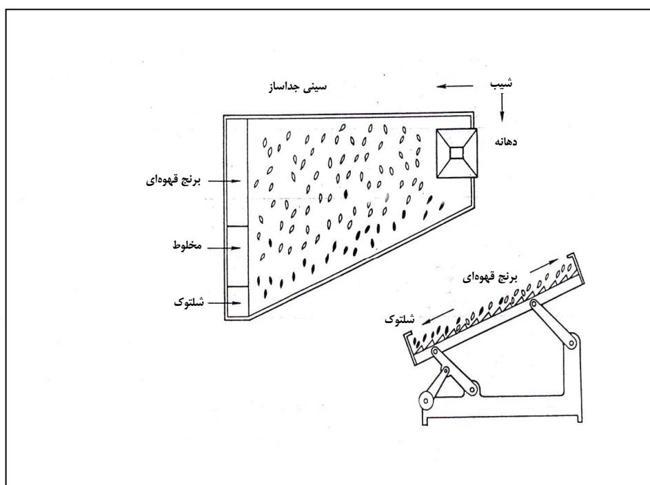
شکل ۱- دستگاه جداساز سینی شکل
