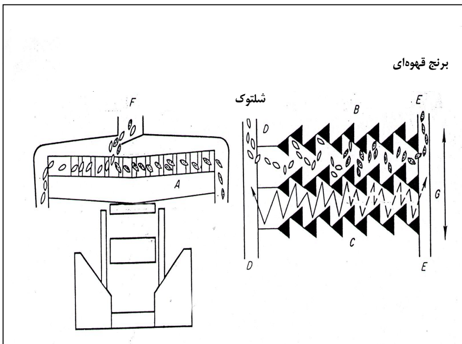
شکل ۲- دستگاه جداساز صندوقی
