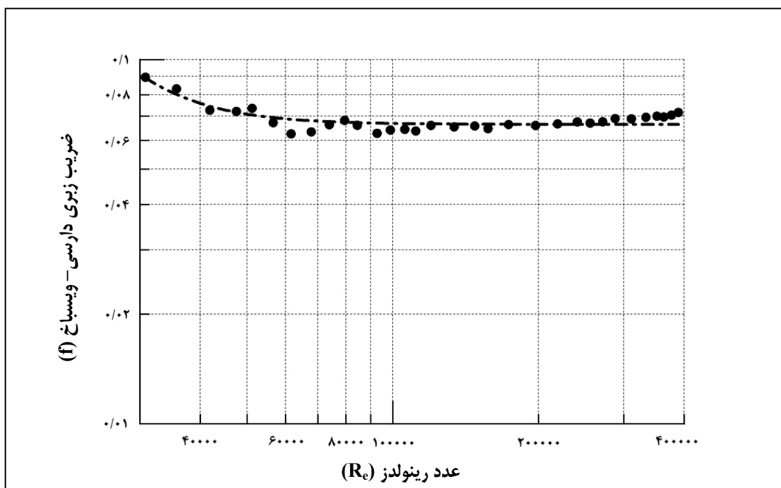
شکل شماره ۴- منحنی تغییرات ضریب زبری دارسی - ویسباخ با عدد رینولدز برای لوله با قطر ۱۱۵ میلی متر
