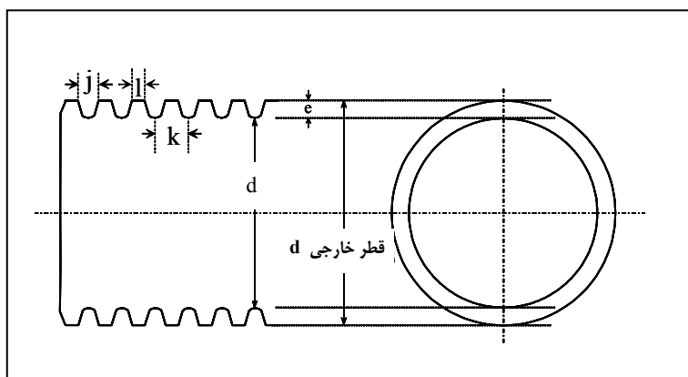
شکل شماره ۱- علائم به کار رفته در لوله‌های موجدار زهکشی
