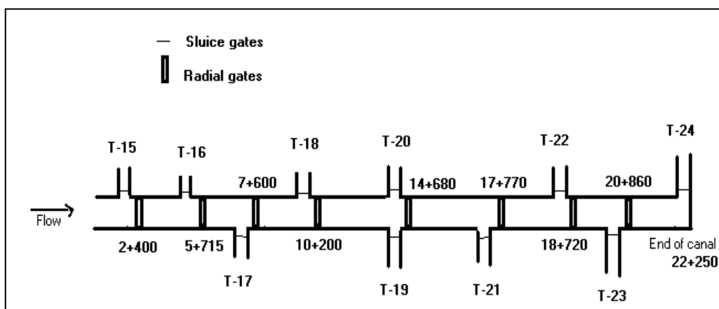
شکل ۳- موقعیت سازه‌ها و کانال‌های درجه ۳ کانال اردیبهشت
