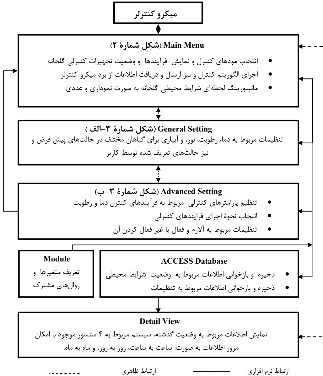
شکل شماره ۱- نمای شماتیک از اجزای نرم افزار کنترل و مانیتورینگ گلخانه
