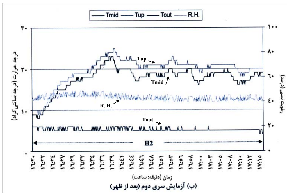
شکل شماره ۶- نتایج آزمایش مربوط به ارزیابی سیستم در کنترل دما. (الف) ساعت ۹:۲۰ تا ۱۰:۴۵ با مدام و (ب) (ب) ۱۶:۲۰ تا ۱۷:۲۰- روز ۱۷ آذر ماه ۱۳۸۲
