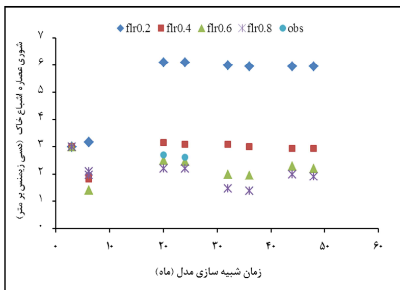
شکل ۳- واسنجی راندمان آبشویی منطقه ریشه
