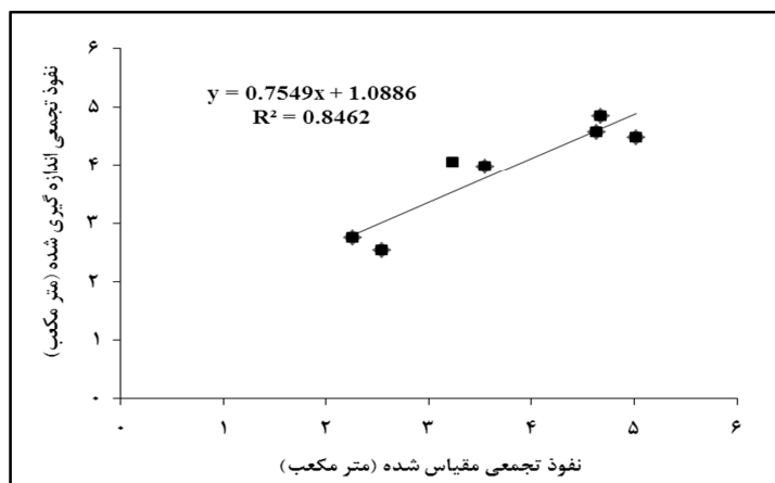
شکل ۲- مقایسه حجم آب نفوذ یافته واقعی و مقیاس شده برای هفت واقعه آبیاری در روش جویچه‌ای یک در میان ثابت
